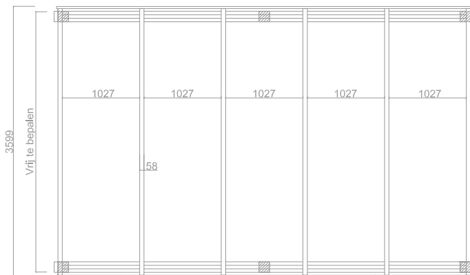
BOVENAANZICHT
