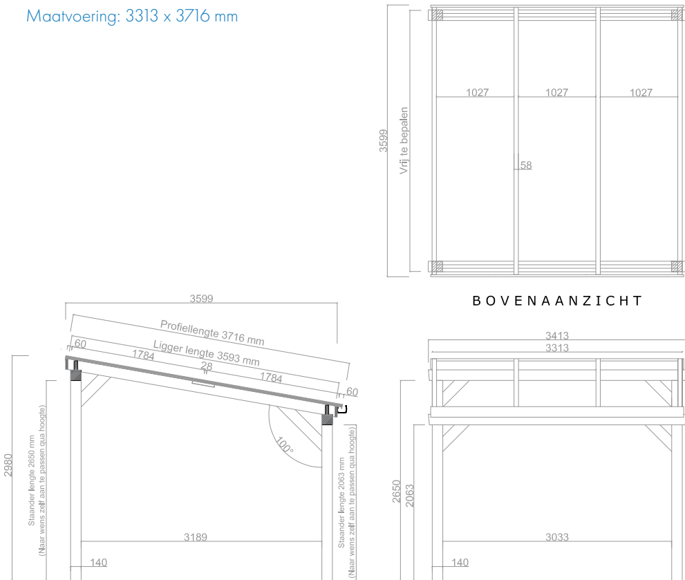
DOORSNEDE
