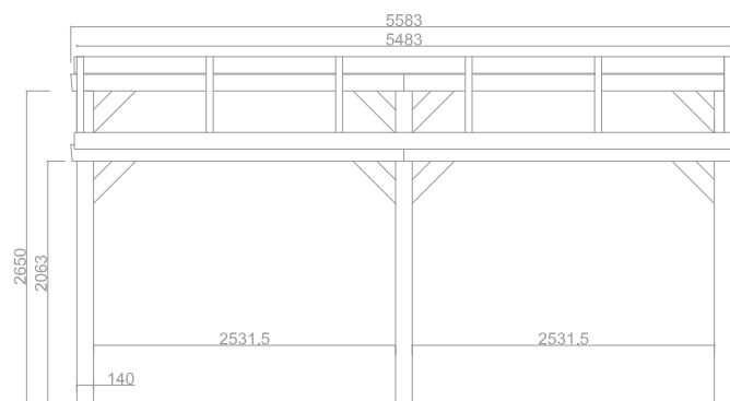
VOORAANZICHT
