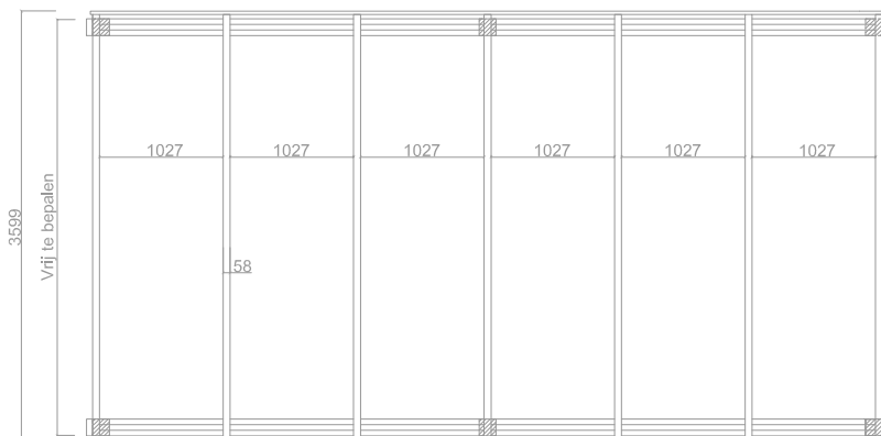
BOVENAANZICHT
