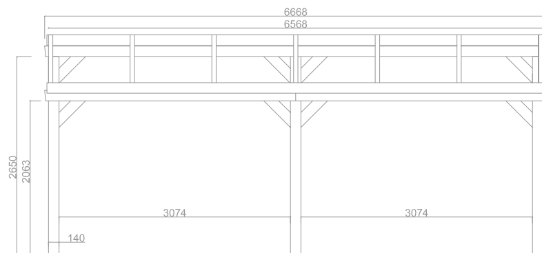
VOORAANZICHT
