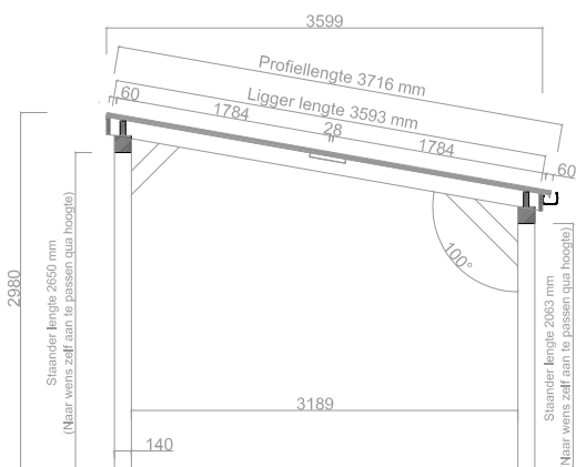
DOORSNEDE
